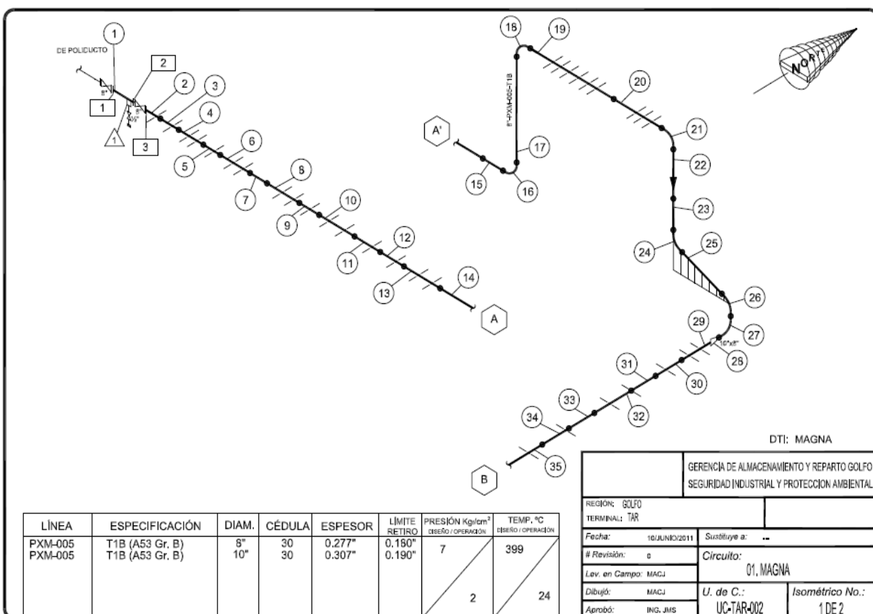
Figura 10. Diagrama isométrico 1 de 2 de la UC-002 del circuito de Magna.
