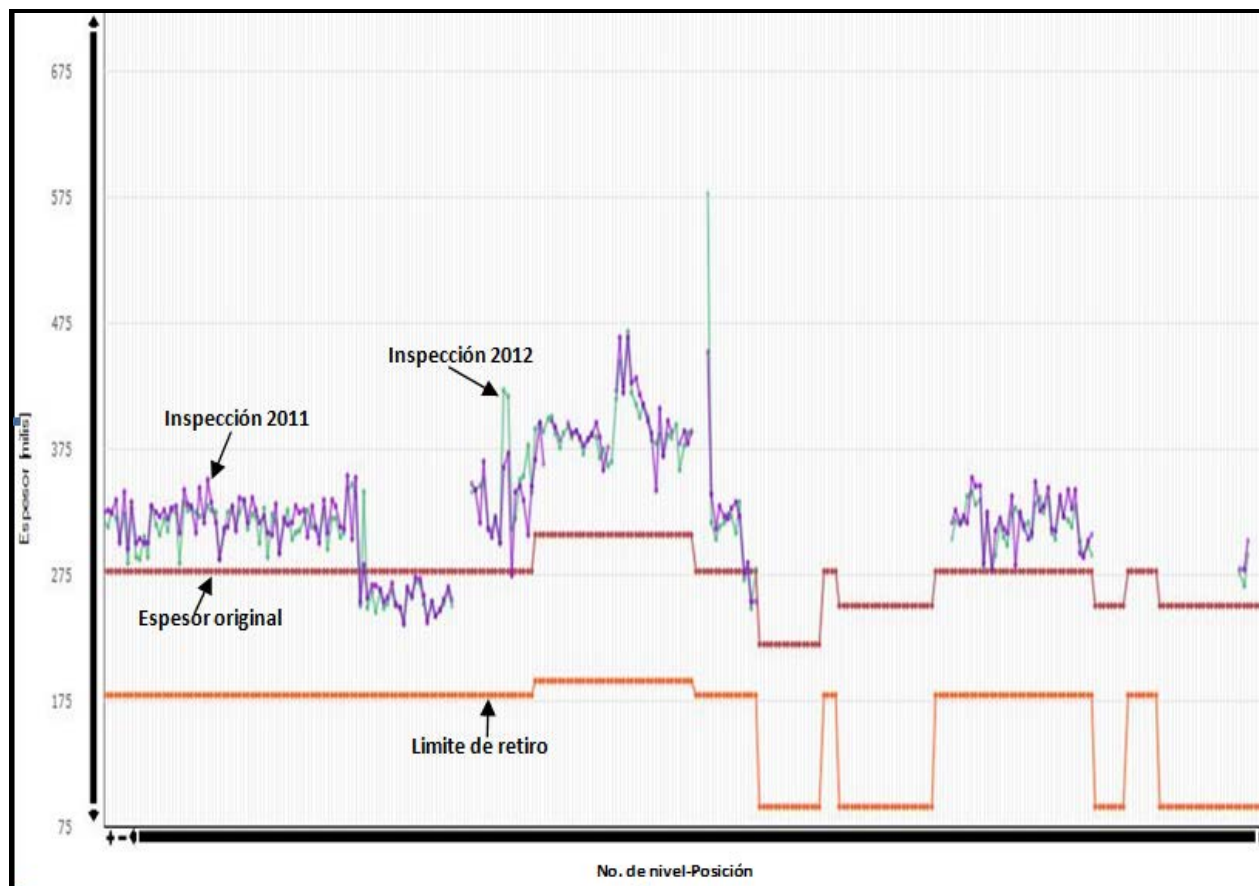
Figura 15 Gráfica de mediciones de espesor.
