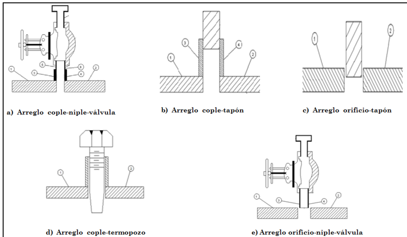
Figura 6. Arreglos típicos de niplería.
