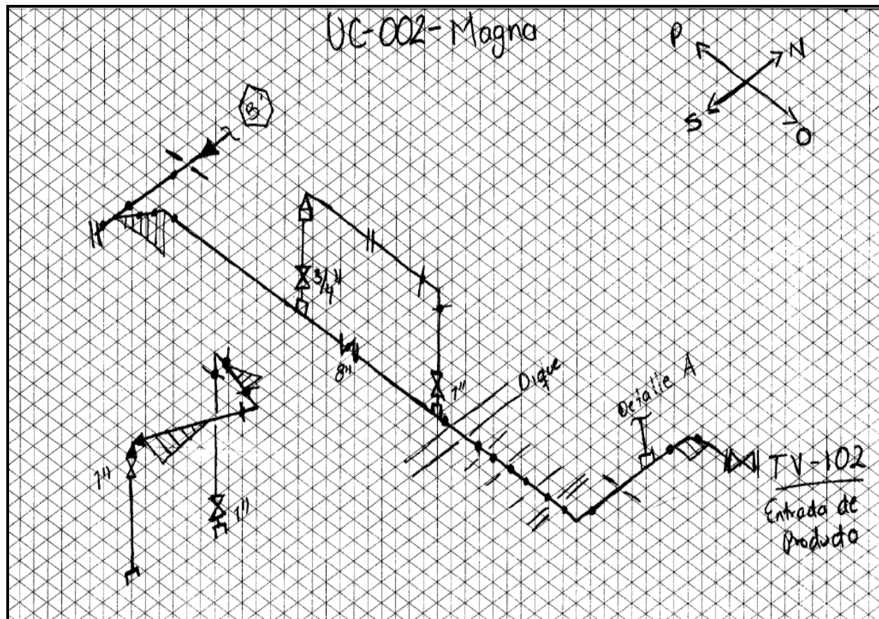
Figura 9. Levantamiento típico en papel isométrico.
