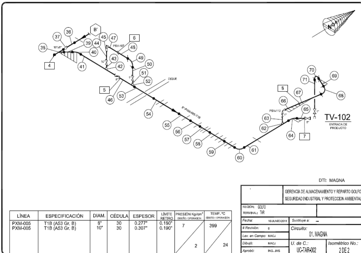
Figura 10.1 Diagrama isométrico 2 de 2 de la UC-002 del circuito de Magna.
