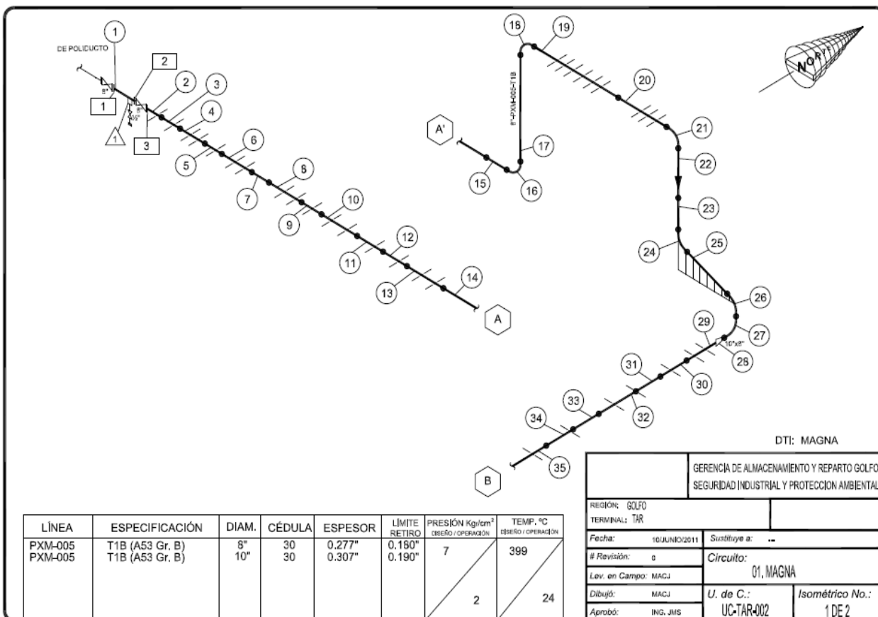
Figura 5. Niveles de tubería, nipleria y tornillería señalados en un diagrama isométrico.
