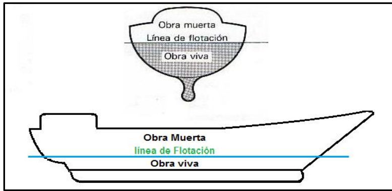
Figura 4-16 Obra muerta, obra viva y líneas de flotación del casco de un buque. ( nauticajonkepa.wordpress.com )
