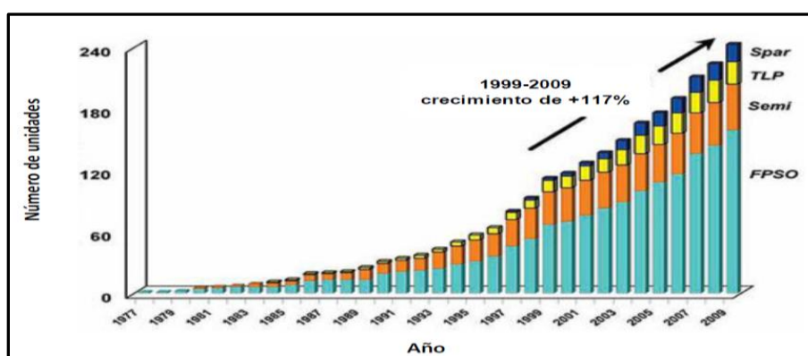
Figura 4-43 Incremento en el uso de Sistemas flotantes de producción en el mundo de 1977 a 2009. (Barranco, 2012)
