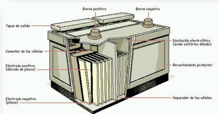
Figura 1.18 Batería Plomo/Ácido. Fuente: http://www.electricasas.com
