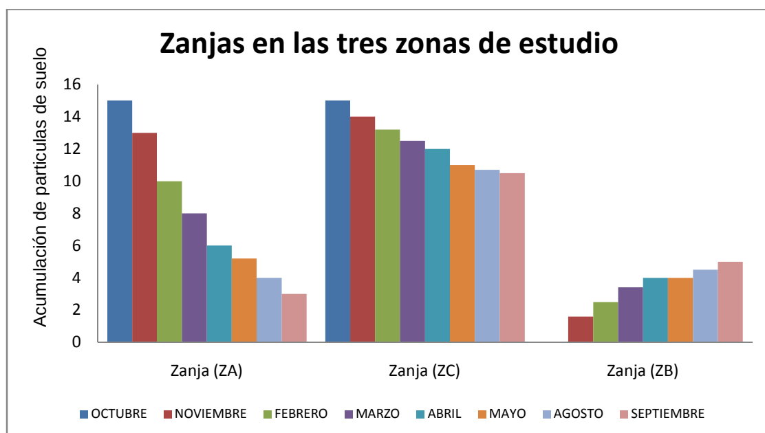
Figura. 16 Acumulación de materiales disgregados (clastos) en las zanjas de las tres zonas de estudio
