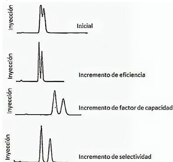
Figura 4. Importancia de cada parámetro en la resolución de un cromatograma 10
