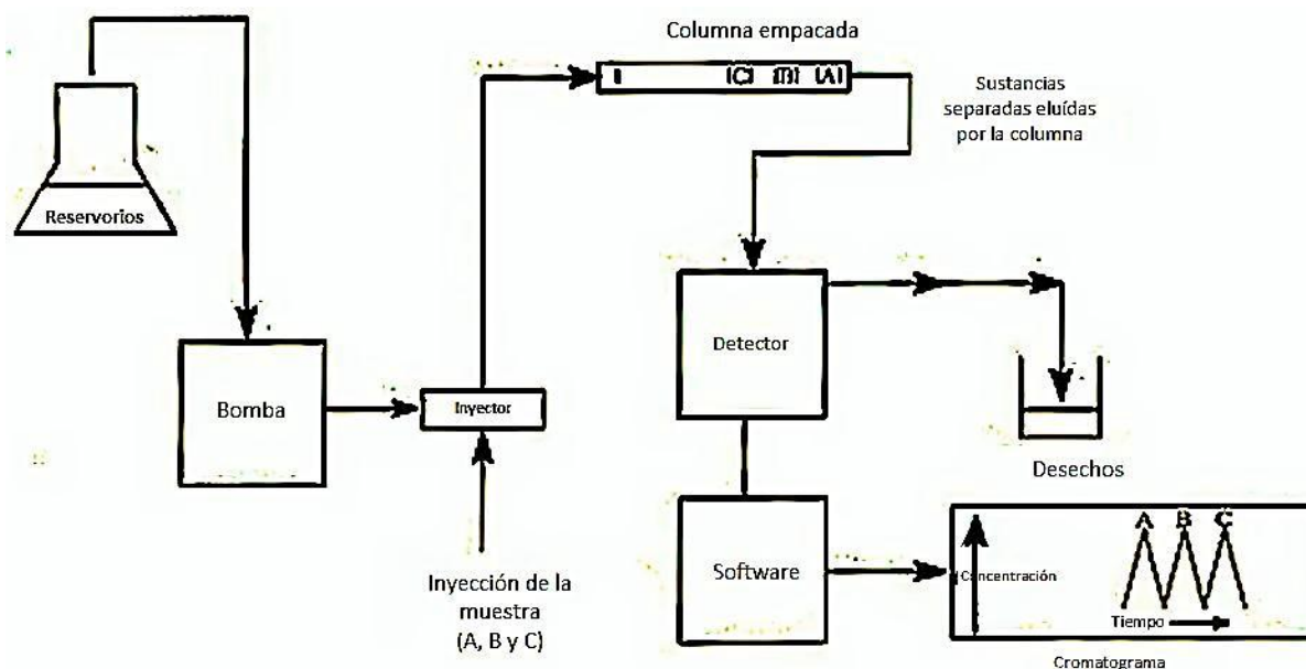
Figura 5. Componentes generales de un instrumento para CLAR 16
