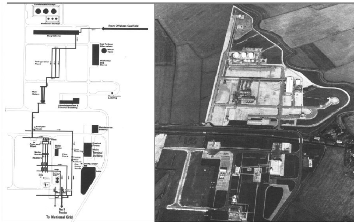
Figura 7. Plano de Localización General.
