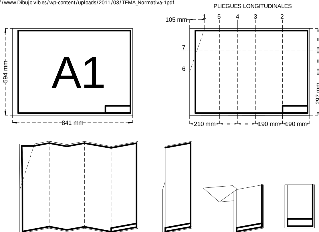
Figura 10. Doblado del formato A1.
