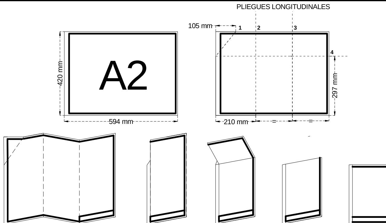
Figura 9. Doblado del formato A2.
