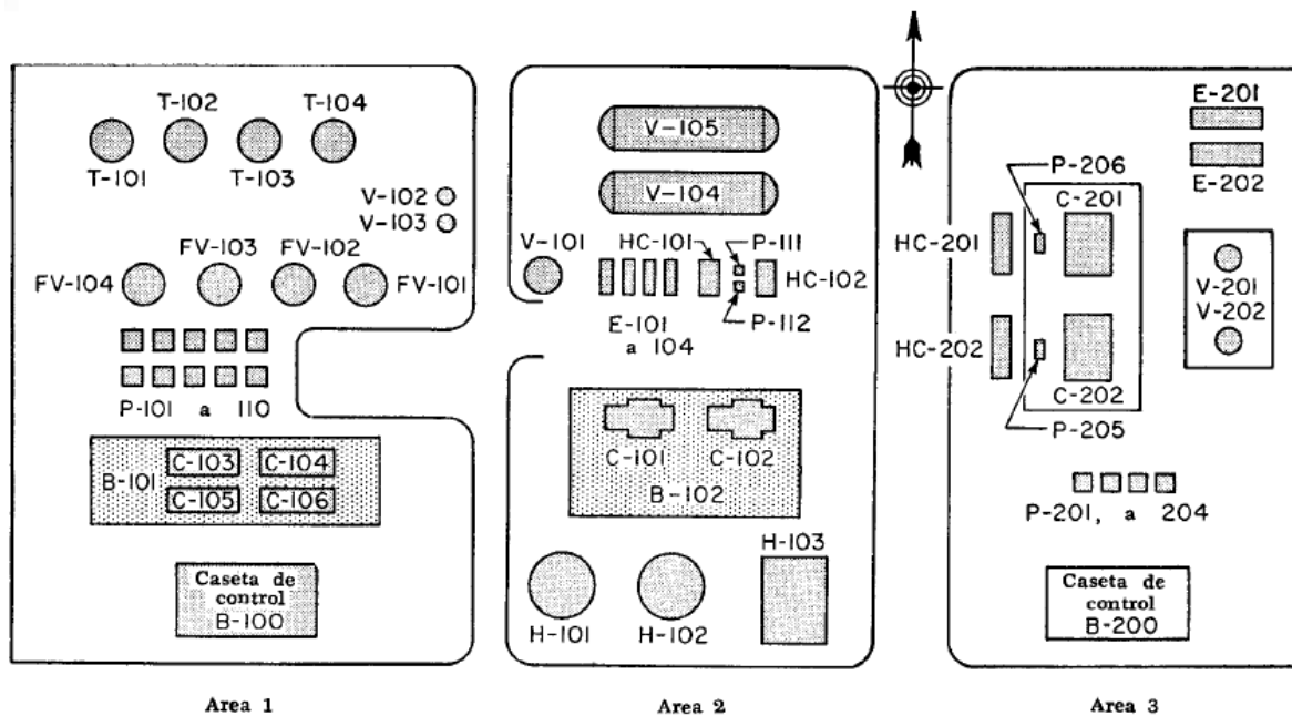
Figura 6. Plano de Localización General de Equipo.
