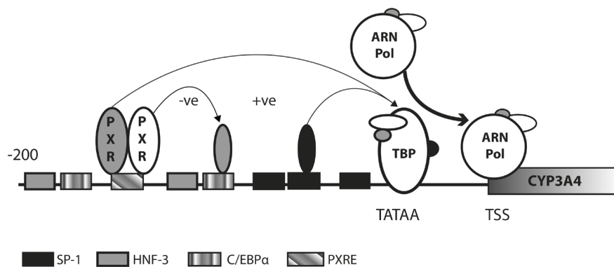
Figura 7.5. Elementos involucrados en la expresión del gen CYP3A4 mediada por xenobióticos (Modificado de Plant, 2003).
