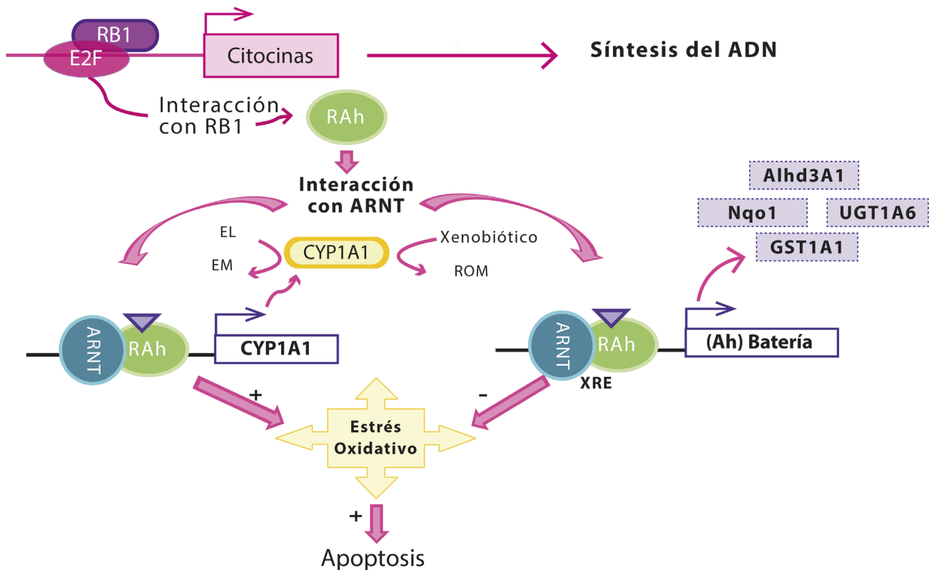
Figura 5.5. Papel del RAh en la señalización celular (Modificado de Plant, 2003).
