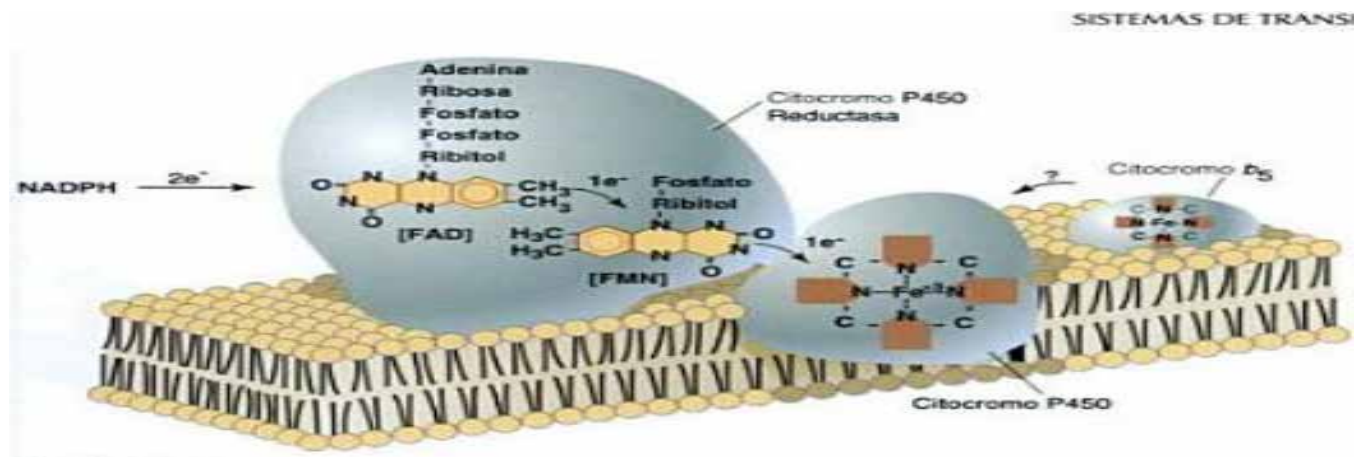
Figura 2.7. Componentes del Citocromo P450 (Miwa et al. , 1979; Devlin, 2004).
