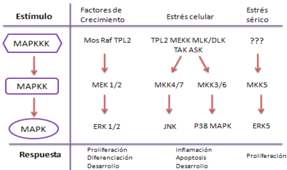
Figura 4.3. Cascada MAPK cinasas en mamíferos (Modificado de Plant, 2003).
