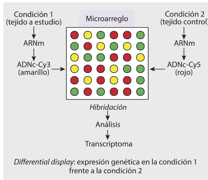
Figura 6.3. Técnica de Microarreglos (Busquets y Agusti, 2001).
