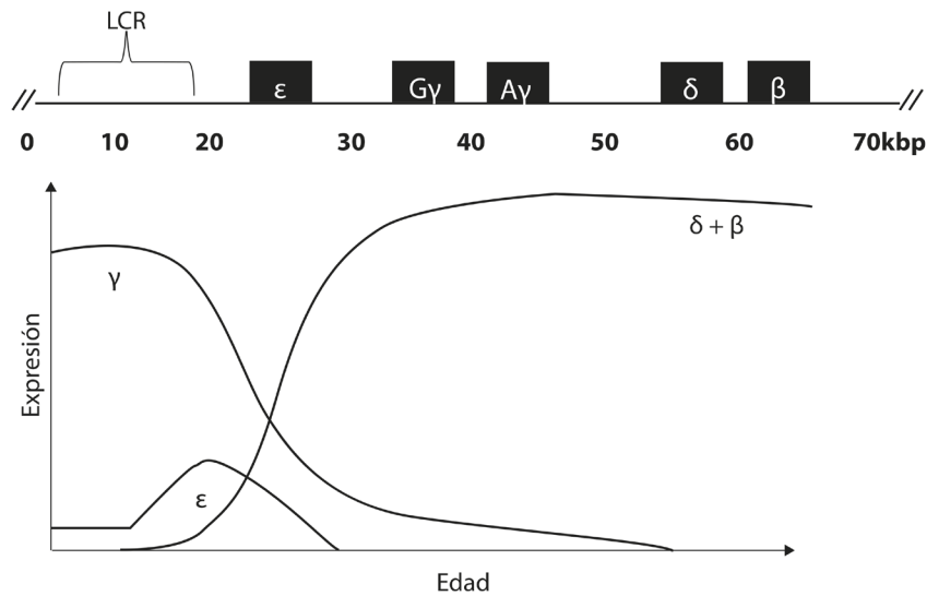
Figura 7.3. El grupo de genes humanos \beta -globulina (Modificado de Plant, 2003).
