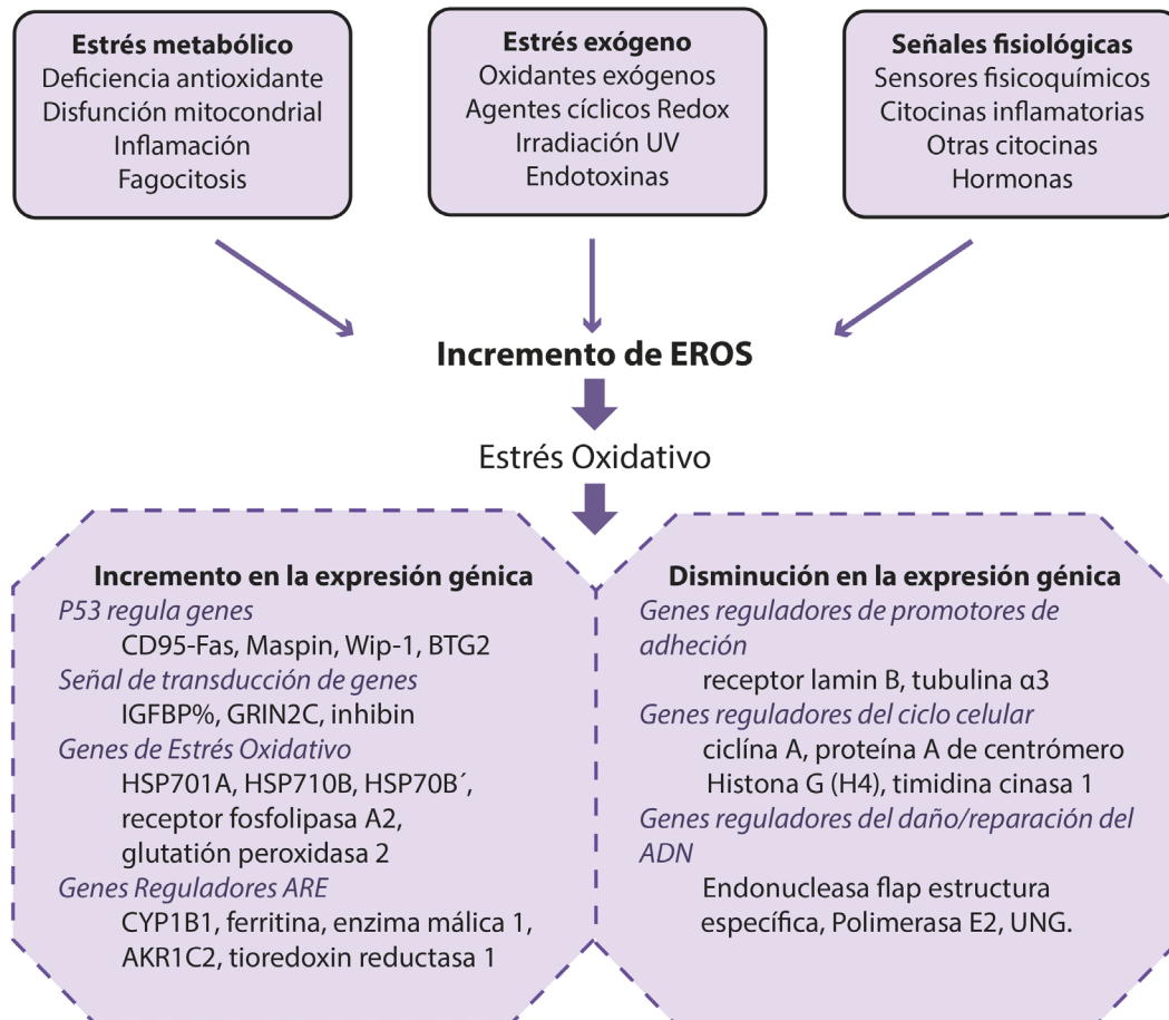
Figura 4.4. Cambios en la expresión génica causados por EROS (Modificado de Plant, 2003).
