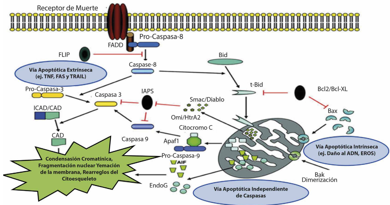
Figura 4.7. Vías de inducción de apoptosis (Modificado de Ghavami et al. , 2009).
