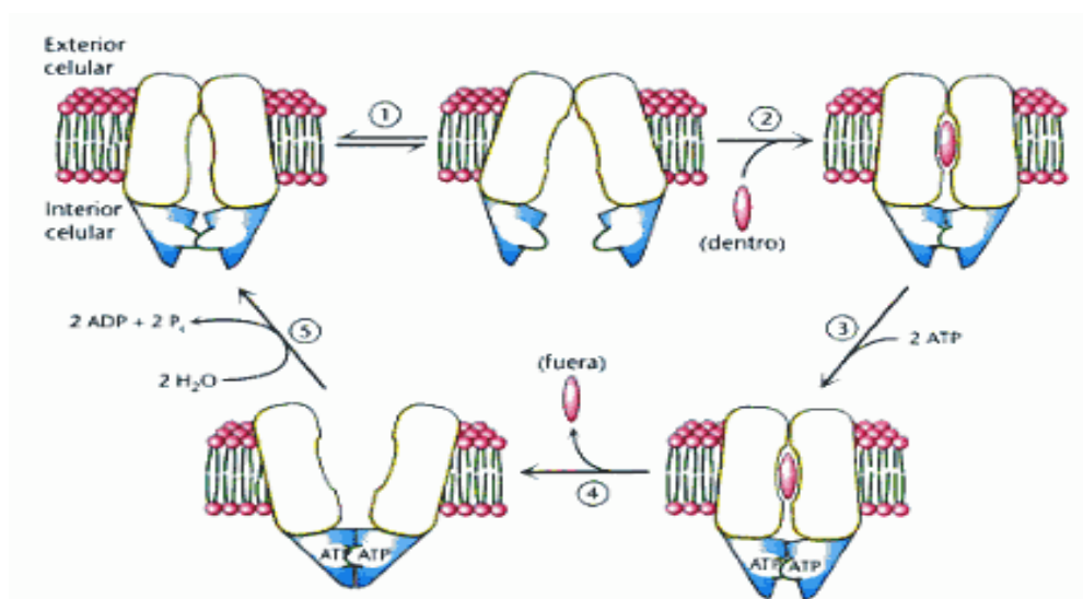
Figura 1.2. Mecanismo de un transportador ABC. 1. Apertura del conducto hacia el interior de la célula; 2. Fijación del sustrato y cambio conformacional; 3. Unión del ATP y cambios conformacionales consiguientes; 4. Separación de los dominios que separan la membrana y liberación del sustrato al otro lado de la membrana; 5. Hidrólisis del ATP y restauración del transportador en su estado inicial (Mendoza, 2008).
