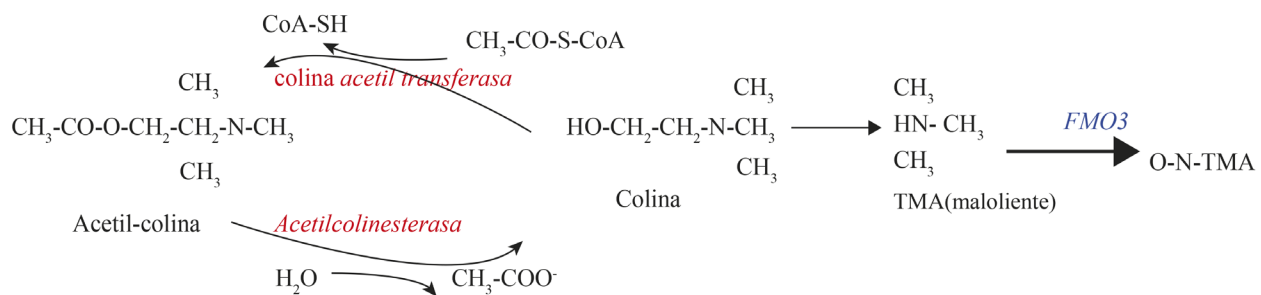
Figura 2.4. Toxicidad mediada por la MOF3 de la TMAuria (Treacy et al. , 1998).
