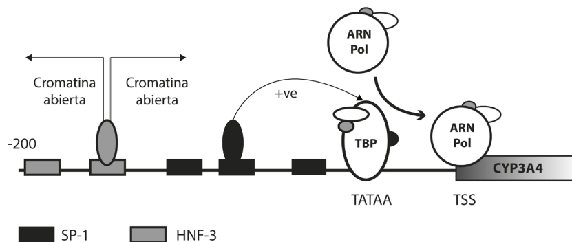
Figura 7.4. Elementos involucrados en la expresión constitutiva del gen CYP3A4 (Modificado de Plant, 2003).
