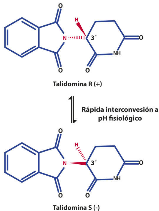
Figura 5.6. Enantiomeros de la molécula de Talidomida (Modificado de Franks et al. , 2004).
