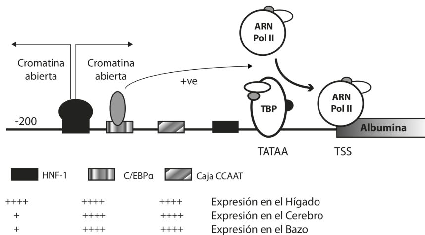
Figura 7.2. Elementos involucrados en la expresión tejido-específica del gen de la Albúmina (adaptado de Lichtsteiner et al. , 1987).
