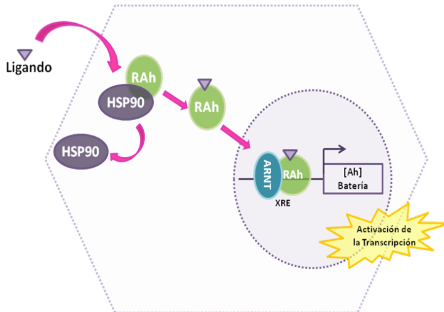
Figura 5.4. Activación de la transcripción de genes en batería (Modificado de Plant, 2003).
