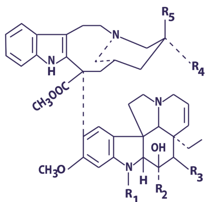
Figura 5.1. Estructura general de Alcaloides de Vinca : Vincristina, Vindestina y Vinblastina (Jordán et al. , 1991).
