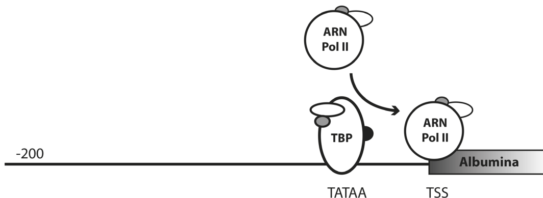
Figura 7.1. Elementos involucrados en la expresión basal del gen de la Albúmina (Modificado de Plant, 2003).
