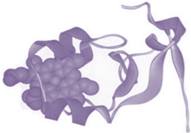
Figura 2.10. Citocromo b5 Reductasa.
