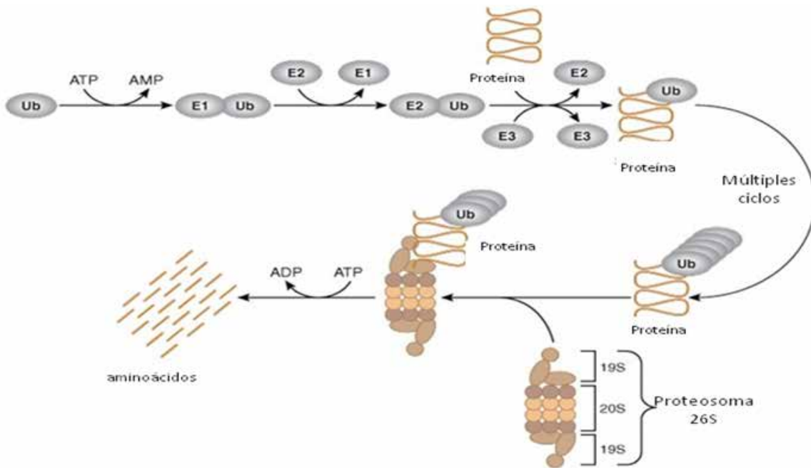
Figura 4.6. Sistema de ubiquitinación para degradación de proteínas (cellsignal.com).
