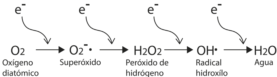
Figura 4.2. Generación de diferentes EROS por la transferencia de energía o reducción univalente secuencial de la formación de especies reactivas no relacionadas en el interior de la célula, formando agua que es fácilmente eliminada (Modificado de Plant, 2003).
