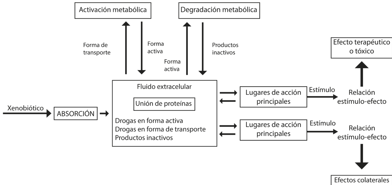
Figura 1.5. Vías Metabólicas (Lauwerys, 1994).
