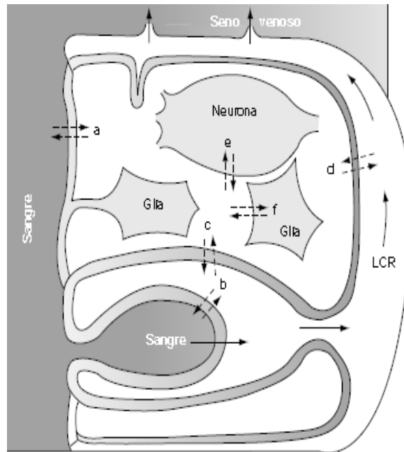
Figura 1.4. Esquema de los compartimentos intracraneales. Las flechas continuas indican la dirección del flujo del líquido cefalorraquídeo.
