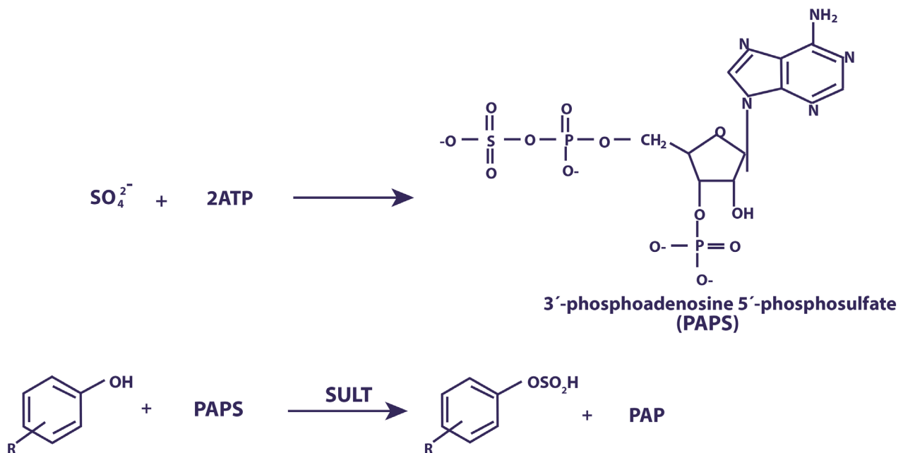
Figura 3.3. Reacción general catalizada por las SULT (Jancova, 2010).
