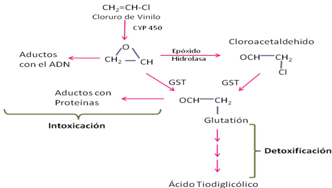
Figura 5.2. Toxicidad del cloruro de vinilo (Modificado de Plant, 2003).
