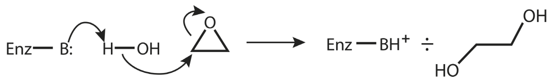
Figura 3.4. Catálisis general por hidratación directa del epóxido (Liang et al. , 2005).
